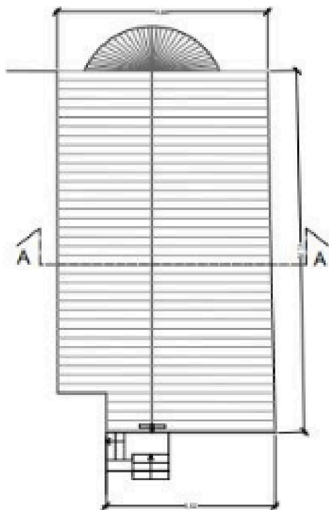
PIANTA COPERTURE
