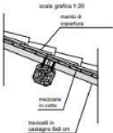
PARTICOLARE DELLA SEZIONE SOLAIO DI COPERTURA
